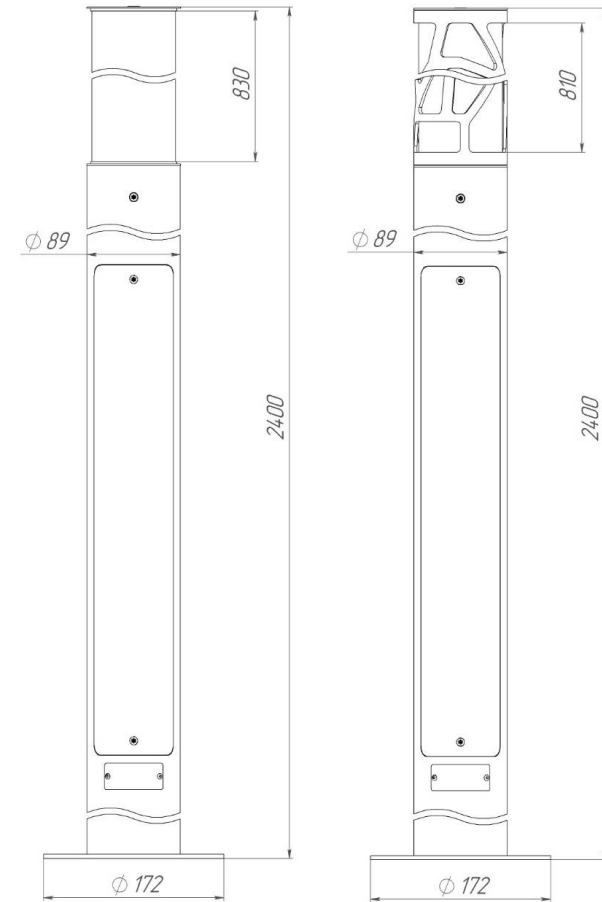
Рисунок 16 Общий вид светильников «L-park PILLAR 2,4», «L-park PILLAR 2,4» спец. исполнение VP
